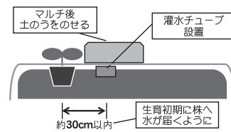
図2 灌水チューブの設置例
